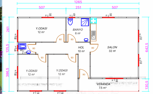
98 m 2 TEK KATLI EV PLANI
