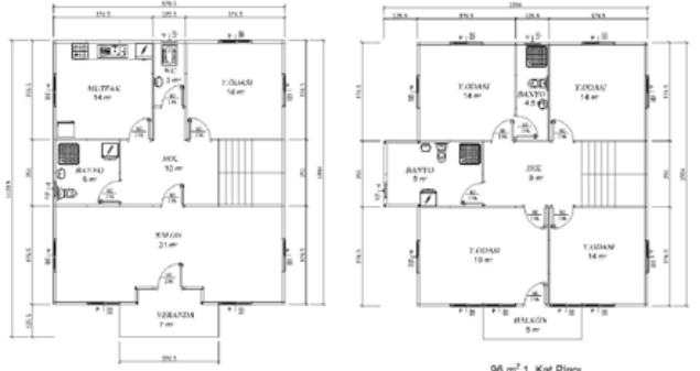
93 m 2 Zemin Kat Planı
