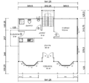
85 m 2 Zemin Kat Planı
