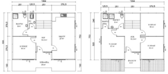
29 + 73 93 m 2 DUBLEKS EV ZEMİN KAT PLANI
