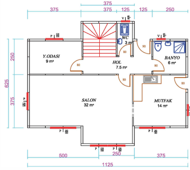
80 m2 DUBLEKS EV ZEMİN KAT PLANI
