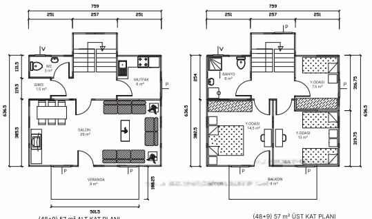
114 m 2 PREFABRİK BİNA PLANI
