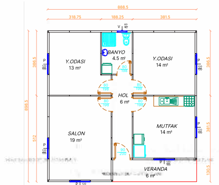
80 m 2 Prefabrik Ev Planı
