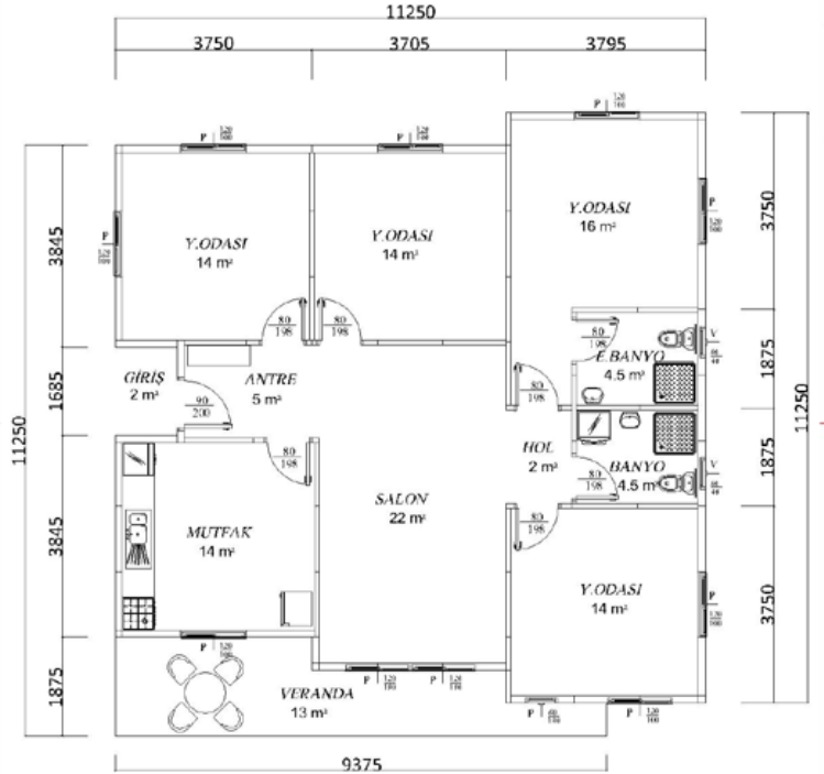
128 m 2 TEK KATLI HAFİF ÇELİK KONSTRÜKSİYON EV PLANI
