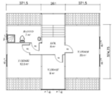
64 m2 DUBLEKS EV ÜST KAT PLANI
