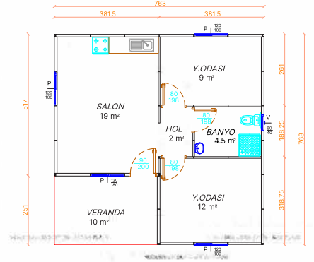
59 m 2 Prefabrik Ev Planı
