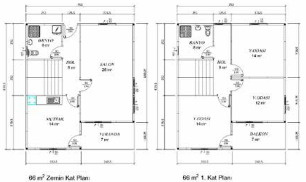
132 m 2 Dupleks Prefabrik Ev Planı
