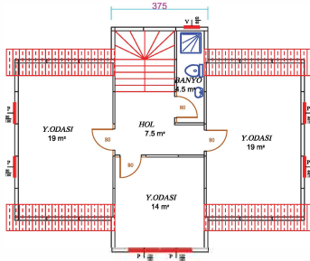
74 m2 DUBLEKS EV ÜST KAT PLANI
