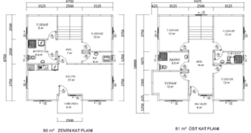
161 m 2 HAFF ÇELİK KONSTRÜKSİYON DUBLEK EV PLANI
