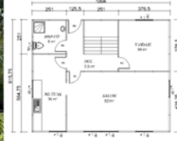
82 m2 DUBLEKS EV ZEMİN KAT PLANI
