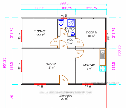
23 + 63 86 m 2 TEK KATLI EV PLANI
