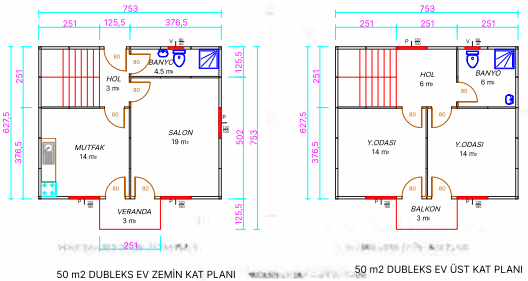
100 m 2 PREFABRİK DUBLEKS EV PLANI
