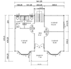
78 m 2 1. Kat Planı
