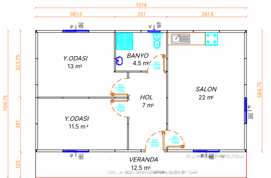
71 m 2 Prefabrik Ev Planı
