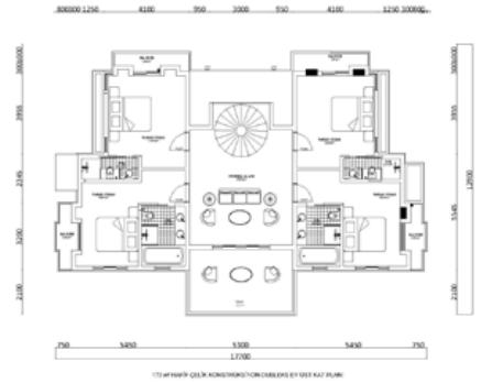
337 m 2 HAFİF ÇELİK KONSTRÜKSİYON DUBLEKS EV PLANI
